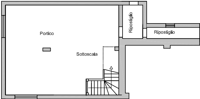
PIANO TERRA h = 2,70 m Superficie utile piano terra: 71.40 mq (escluso portico e scala)
