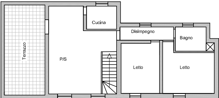
PIANO PRIMO h = 2,70 m Superficie utile piano primo: 89.30 mq (escluso terrazzo)
